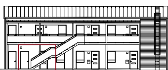
ENTRÉFASAD - ÖST
